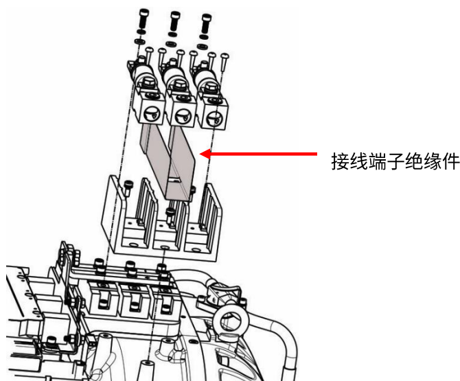
图 1 - 接线端子绝缘件
