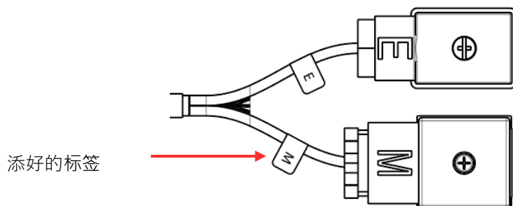
图 2 - 电磁线圈线束标识标签
